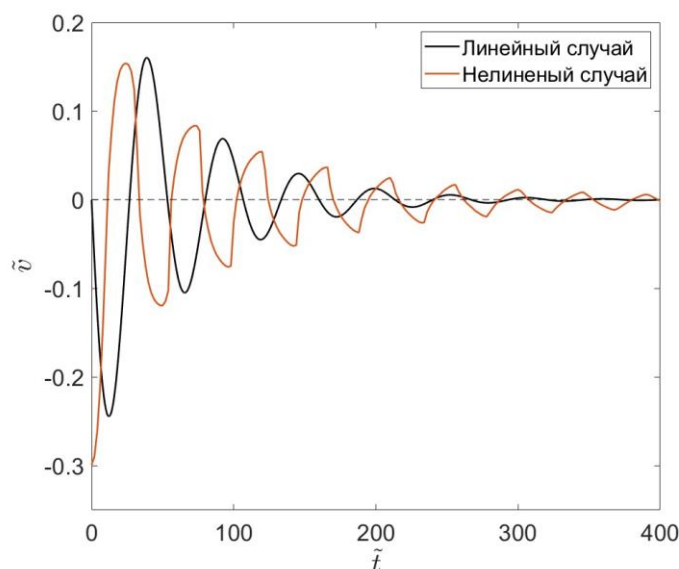
Рисунок 6 – Колебание петли № 6. Figure 6 – Oscillation of loop No. 6.
