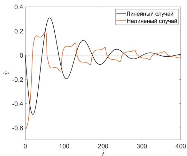
Рисунок 7 – Колебание петли № 7. Figure 7 – Oscillation of loop No. 7.
